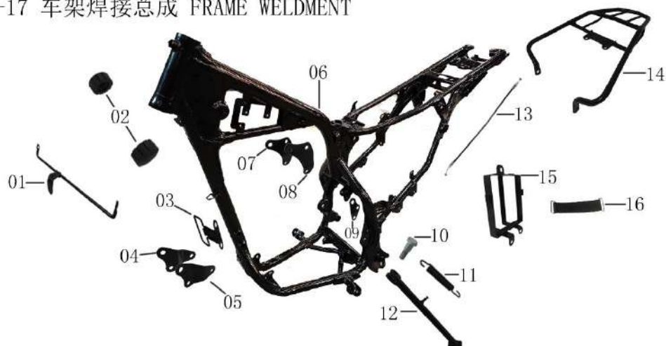
F-17 车架焊接总成 FRAME WELDMENT
